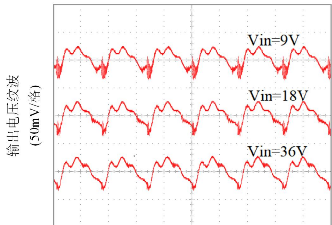
时间 (2μs/格)
