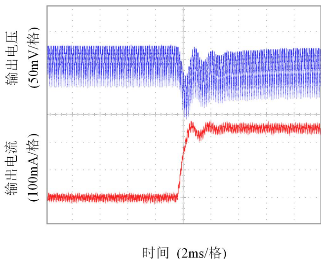
图 5 动态响应
