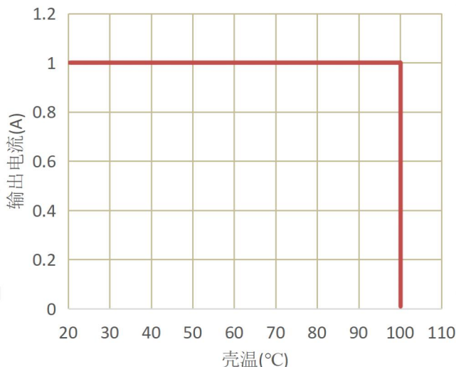
图 6 降额曲线
