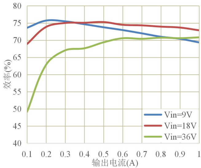
图1 效率 VS 输出电流, T_A=25^{\circ}\text{C}
